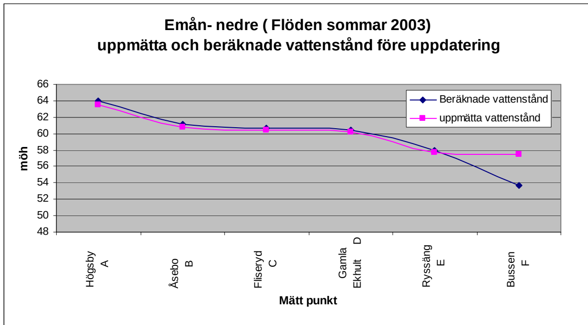
Figur 7. Uppmätt och beräknat vattenstånd i meter över havet (möh) med den hydrauliska modell som har tagits fram under den översiktliga översvämningsskarteringen.
