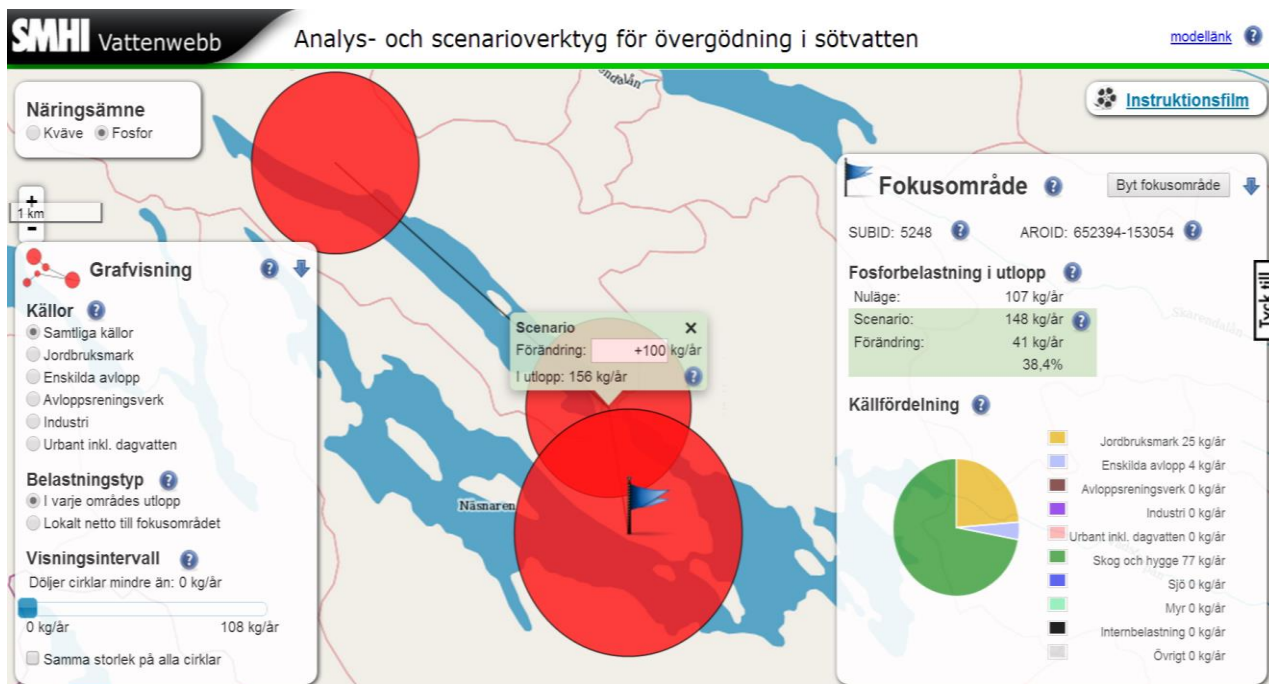
Figur 15. Simulerad effekt av en ökad fosforbelastning i inloppet till sjön Näsnaren. En ökning av 100 kg tot-P/år till sjön ger en nettoökning med 41 kg P/år i utloppet av Näsnaren.
