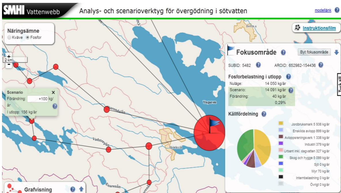
Figur 16. Simulerad effekt av en ökad fosforbelastning i inloppet till sjön Näsnaren. En ökning av 100 kg tot-P/år till Näsnaren ger en nettoökning med 40 kg P/år i utloppet av Yngaren, nästa sjö nedströms.
