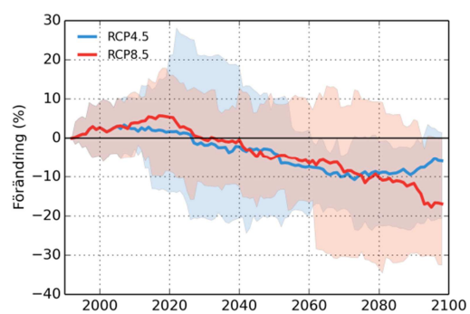
Sangisälven
