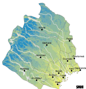
Beräknat 2021-2050
