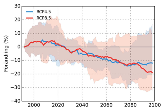
Töreälven
