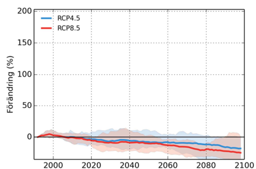
Alterälven
