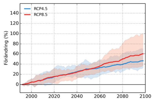
Jämtöälven
