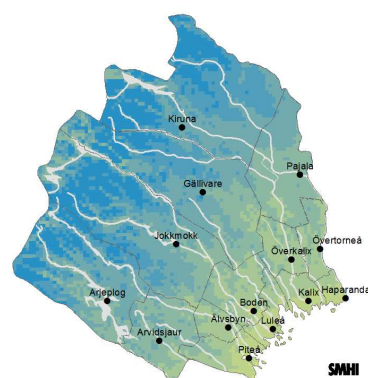
Beräknat 2069-2098
