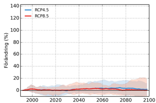
Piteälven
