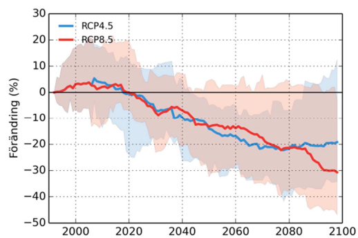
Kalixälven
