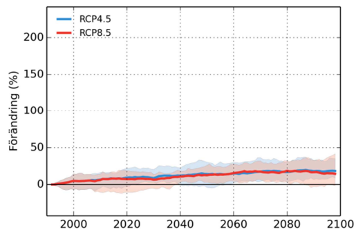
Kalixälven
