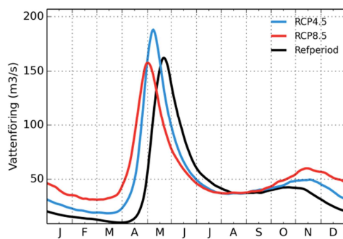
Råneälven
