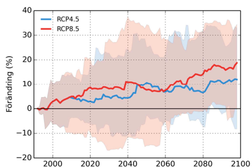
Alån
