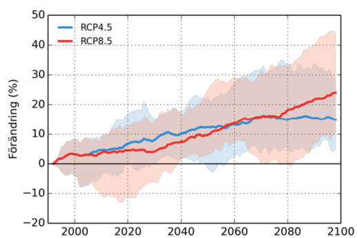
Sangisälven
