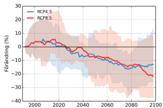
Töreälven
