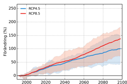
Luleälven, Sitasjaure
