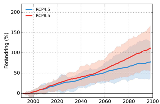
Alån
