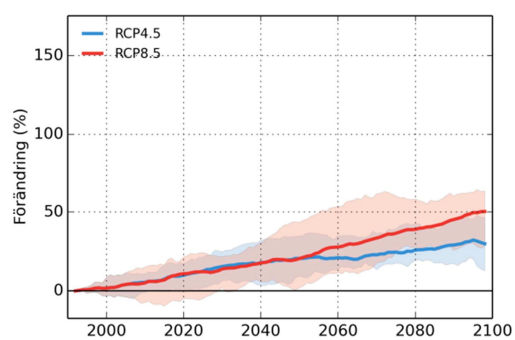
Rosån
