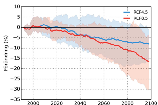
Övre Abiskojoek
