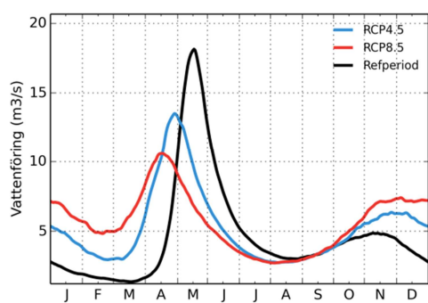
Kalixälven
