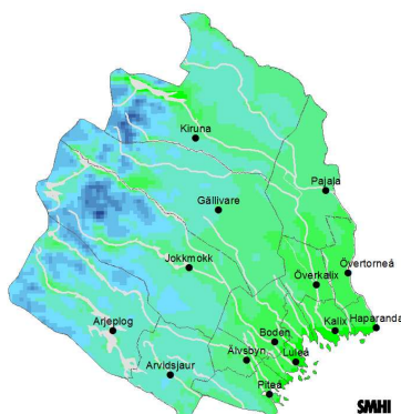
Beräknat 2021-2050
