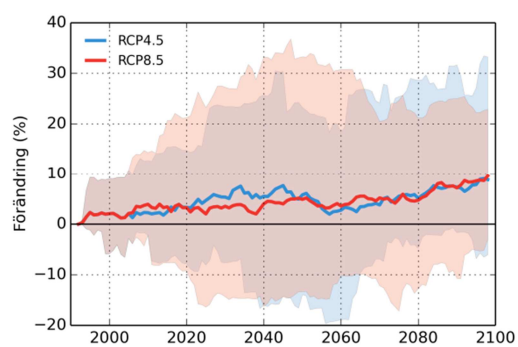
Keräsjoki
