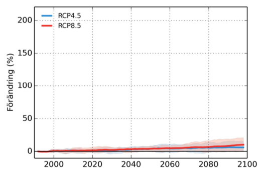
Alån
