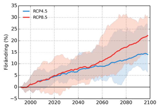
Övre Abiskojokk
