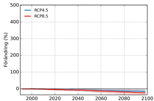
Keräsjoki
