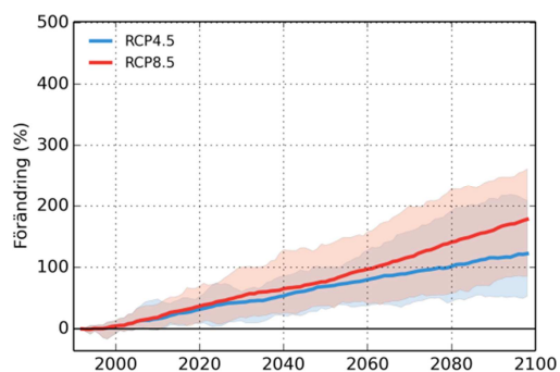
Keräsjöki
