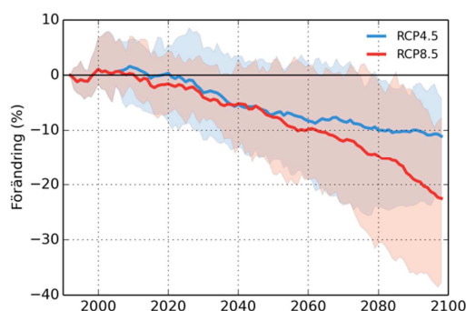
Luleälven, Sitasjaure
