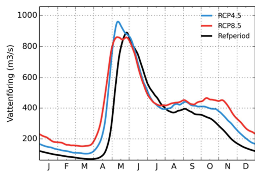
Jämtöälven
