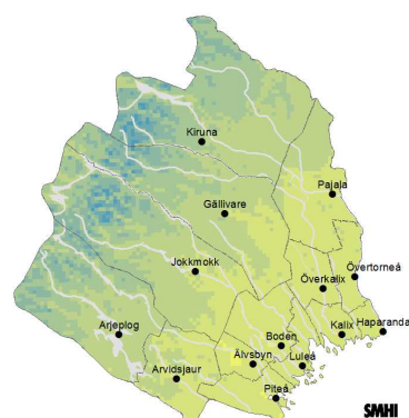
Beräknat 2069-2098
