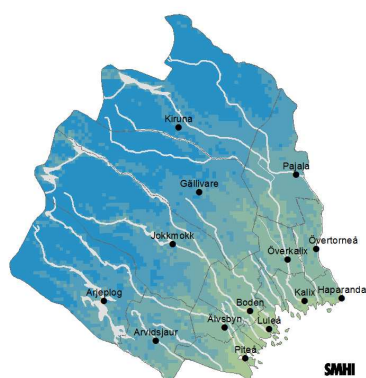
Beräknat 2021-2050
