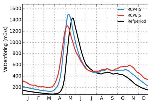
Sangisälven
