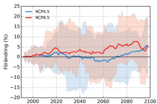
Rosån
