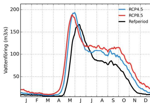
Alån
