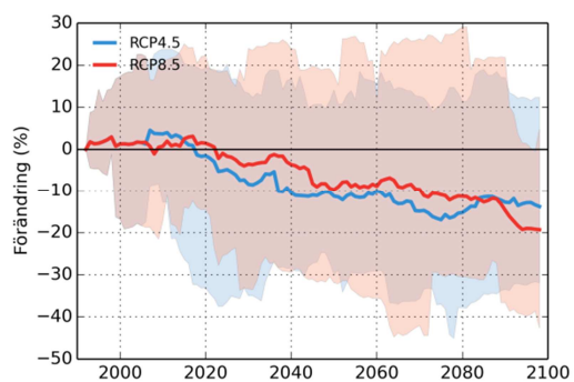
Alterälven
