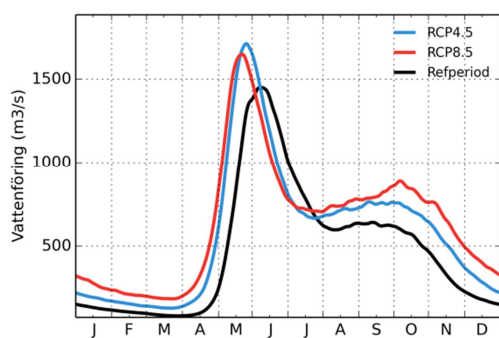
Rosån
