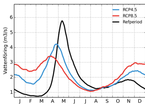
Piteälven
