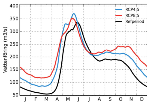
Piteälven
