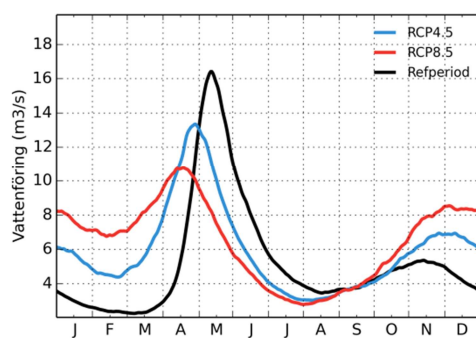
Alterälven
