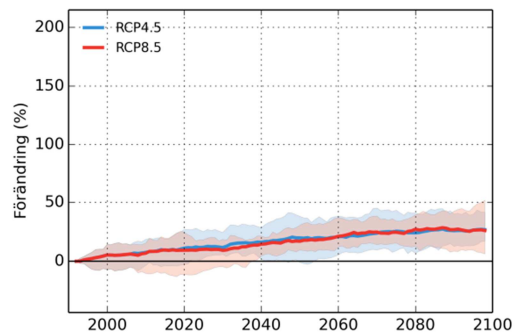
Töreälven
