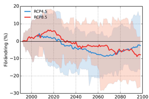
Jämtöälven
