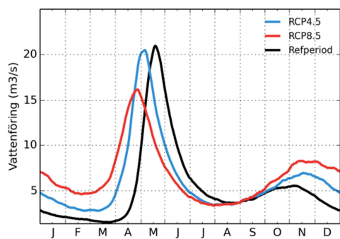
Jämtöälven
