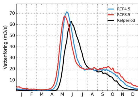
Keräsjoki
