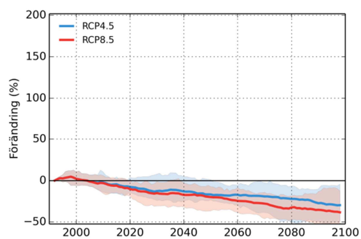
Luleälven
