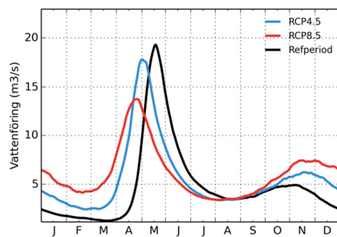
Råneälven
