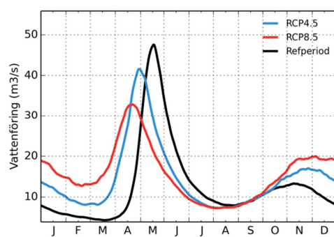
Töreälven
