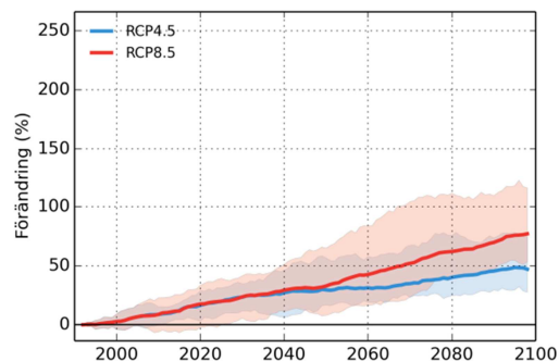
Luleälven, Sitasjaure
