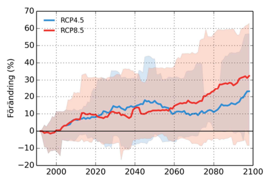
Luleälven, Sitasjaure
