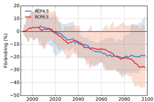
Kalixälven
