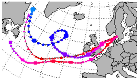
Råö 2010-07-22 18:00
