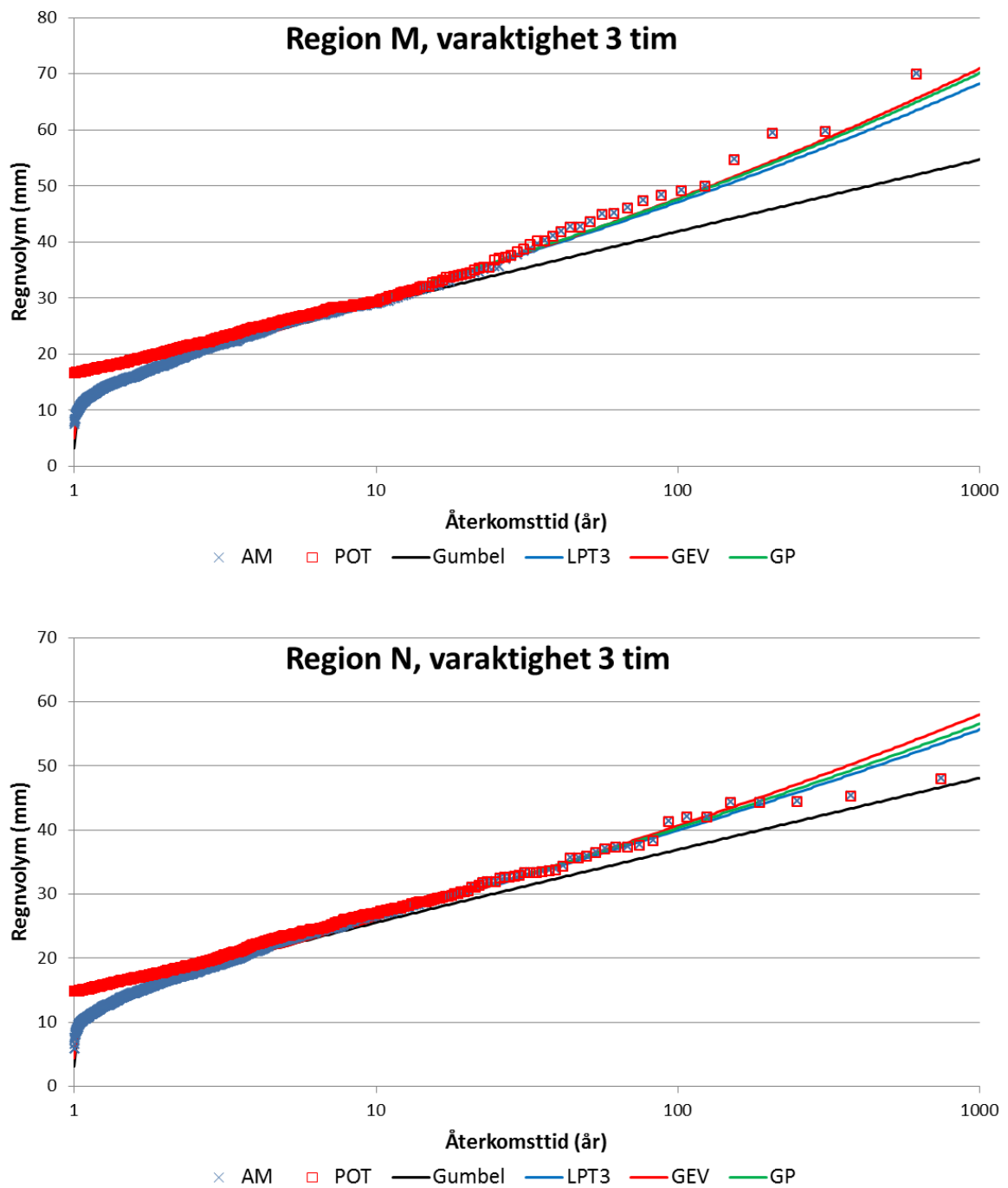
Figur 2. (forts.) Framtagna 3-tim extremvärden och anpassade sannolikhetsfördelningar för de sammanslagna serierna i region M och N.
