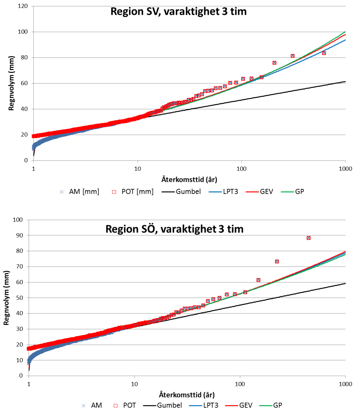
Figur 2. Framtagna 3-tim extremvärden och anpassade sannolikhetsfördelningar för de sammanslagna serierna i region SV och SÖ.
