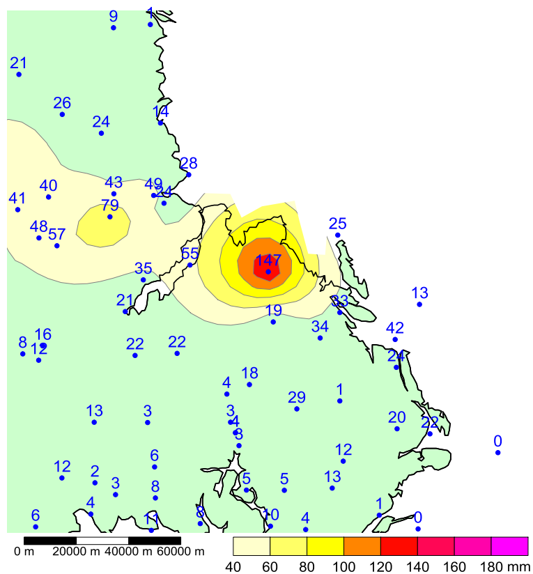
Figur 27. 1989-07-14 - 15 medel nbd 1000 km 2 : 94.6 mm area minst 90 mm: 525 km 2
