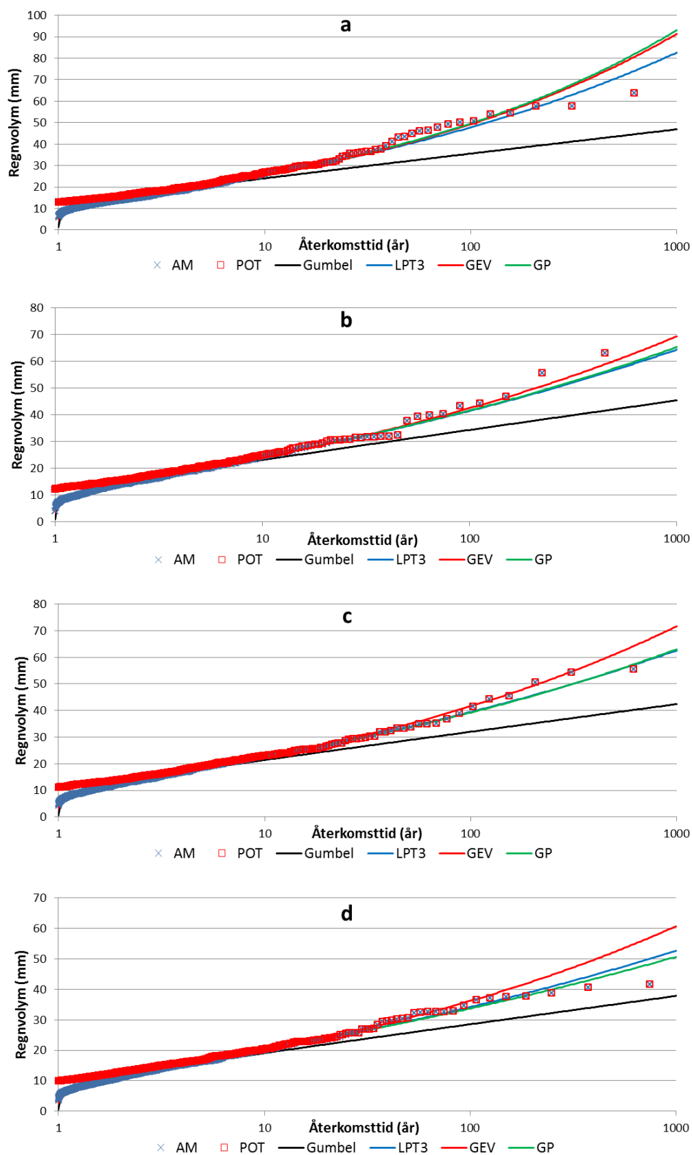
Figur 8. Framtagna 1-tim regnvolymer och anpassade sannolikhetsfördelningar för de sammanslagna serierna i region SV (a), SÖ (b), M (c) och N (d).
