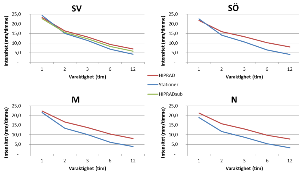
Figur 26. Jämförelse av HIPRAD på 2 \times 2 \text{ km}^2 och 1 tim upplösning med stationsdata för de fyra regionerna för 10-års återkomsttid. Den gröna linjen i region SV exemplifierar hur resultaten påverkas av rumslig sampling, se text.
