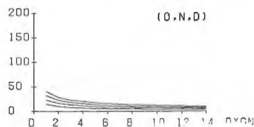
Figur 4.6. Intensitets-varaktighets-frekvensdiagram. Maximal snösmältning och effektiv nederbörd, plottad mot varaktighet för återkomstperioder om 10, 100, 1 000 och 10 000 år (Gumbel-fördelning) för södra Norrland och sydöstra Svealand.
