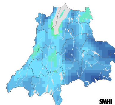
Beräknat 2069-2098
