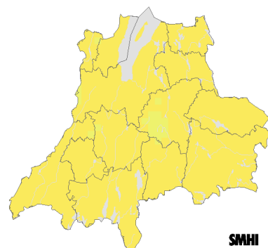
Beräknat 2069-2098
