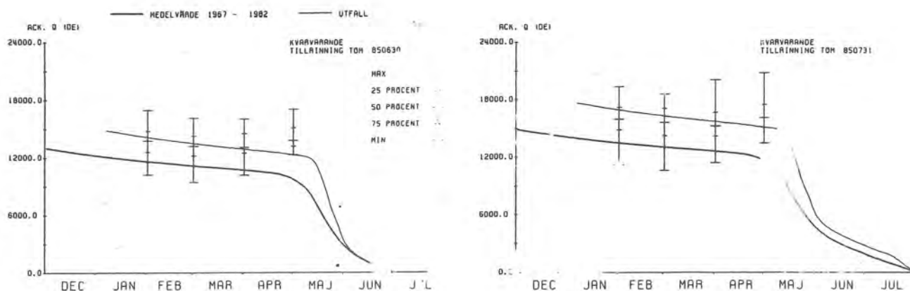
Figur 33. Sammanställning av volymsprognoser med HBV-modellen för Trängslet. Lodräta streck med tvärsreck markerar prognoser med HBV-modellen.
