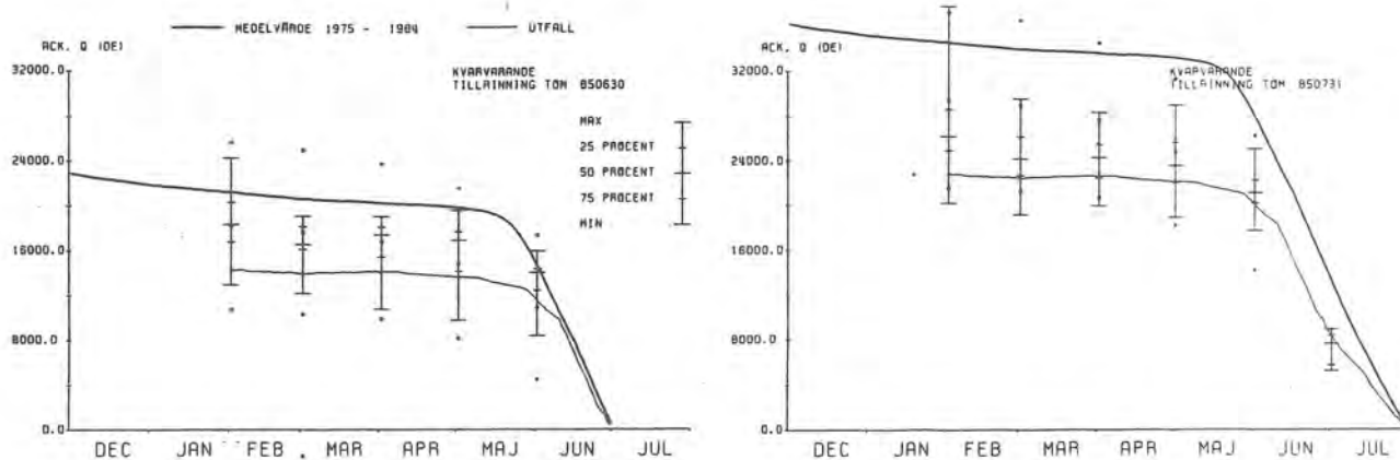
Figur 7. Sammanställning av volymsprognoser för Suorva. Lodräta streck med tvärstreck markerar prognoser med HBV-modellen. Punkter markerar prognoser med arealnederbördsmetoden (10%, 50%, 90%).
