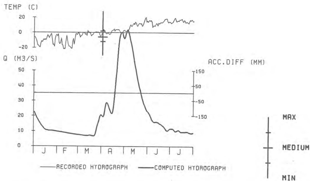
Figur 42. Framkörning av HBV-modellen över vårfloden samt prognos på högsta flödestoppen för Karlslund.
