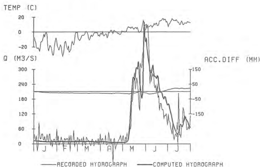
Figur 19. Frankörning av HBV-modellen över vårfloden för Ströms Vattudal
