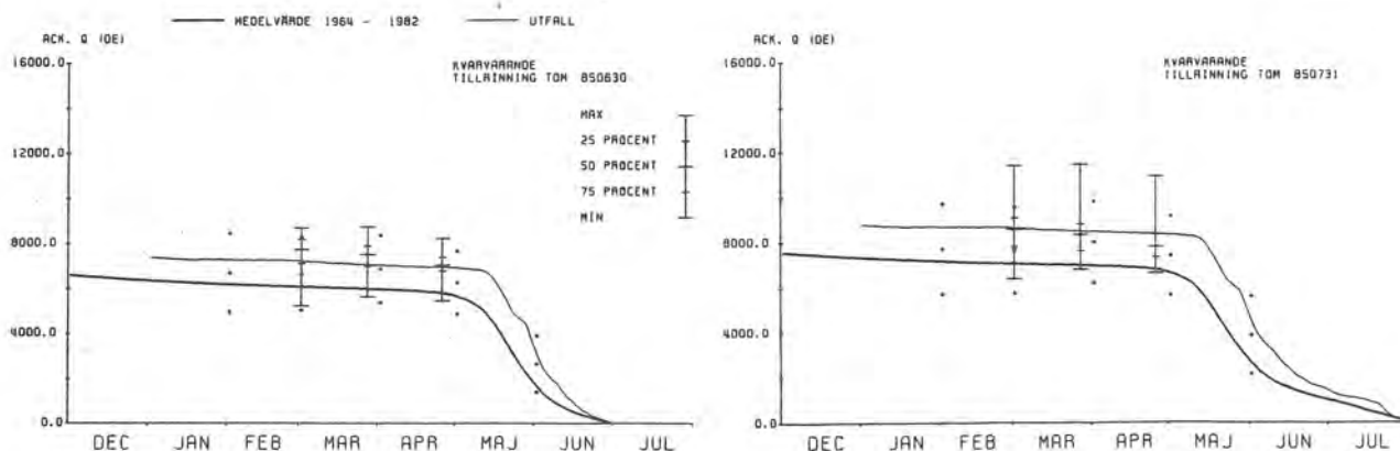
Figur 18. Sammanställning av volymsprognoser för Malgomaj. Lodräta streck med tvärstreck markerar prognoser med HBV-modellen. Punkter markerar prognoser med arealnederbördsmetoden (10%, 50%, 90%).
