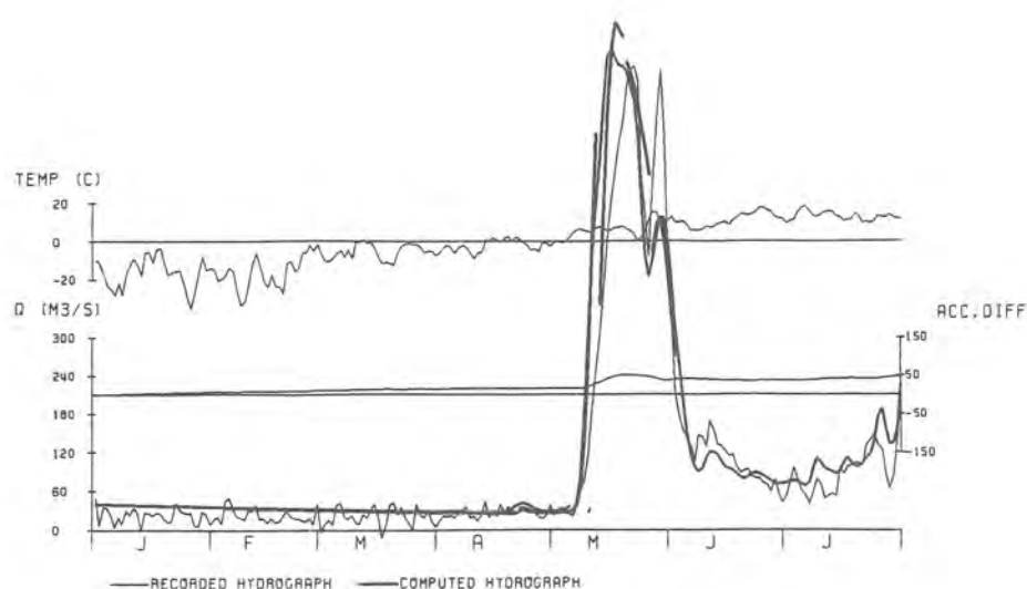
Figur 26. Framkörning av HBV-modellen över vårfloden samt korttidsprognoser för Svegsjön.
