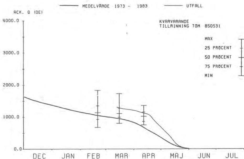
Figur 39. Sammanställning av volymsprognoser med HBV-modellen för Bernshammar. Lodräta streck med tvärstreck markerar prognoser med HBV-modellen.
