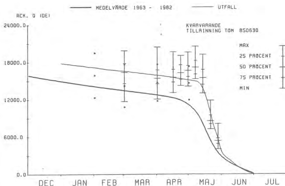
Figur 27. Sammanställning av volymsprognoser med HBV-modellen för Svegsjön. Lodräta streck med tvärstreck markerar prognoser med HBV-modellen. Punkter markerar prognoser med arealnederbördsmetoden (10%, 50%, 90%).
