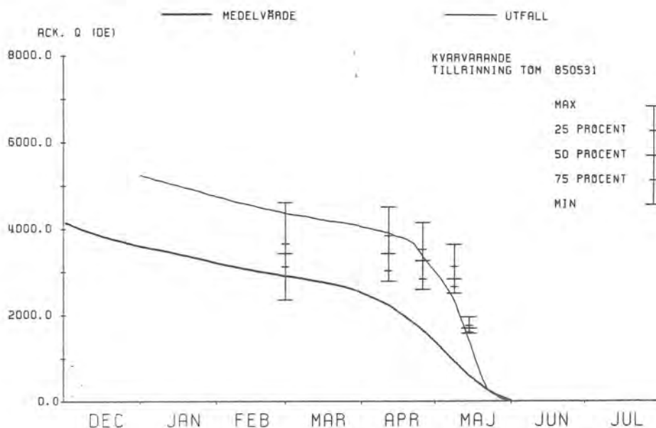
Figur 31. Sammanställning av volymsprognoser med HBV-modellen för Tolvfors. Lodräta streck med tvärstreck markerar prognoser med HBV-modellen.
