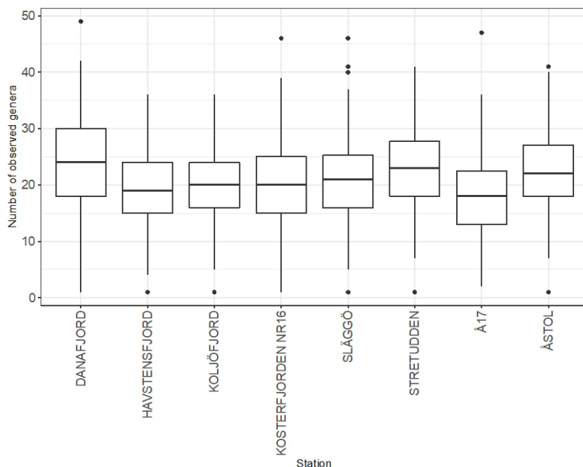
Fig. 29. Box and whisker diagram som visar variationen för antal observerade släkten för hela perioden på 8 utvalda stationer. Helden horisontell linje visar medianvärde, horisontella linjer över och under medianvärdet visar övre (75 %) respektive undre (25 %) kvartilen och det vertikala strecket visar det maximala och minimala värdet. Punkter visar extremvärden eller s.k. outliers.
