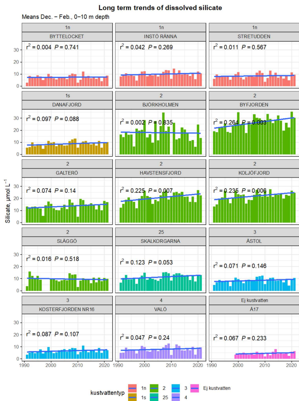
Fig. 44. Koncentration av löst kisel (silikat), se figur 42 för detaljer.
