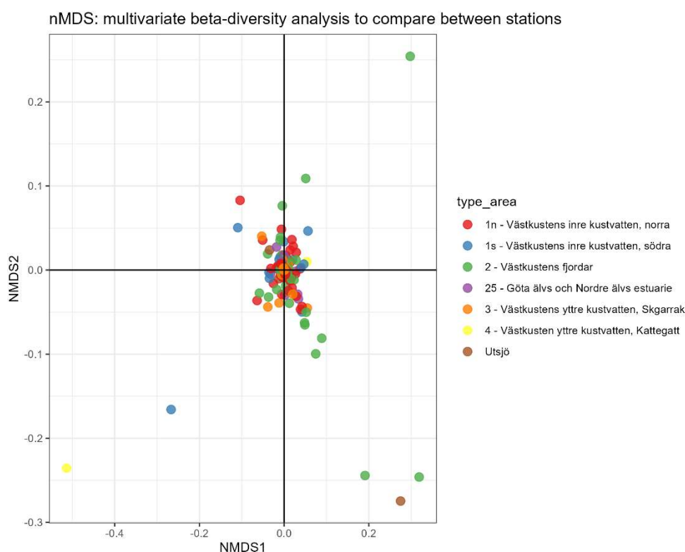
Fig.33. En non-metric multidimensional scaling ordinansanalys (Betadiversitet) som visar skillnader mellan olika planktonsamhällen baserat på data från släkten (genus). Färgerna indikerar typområden. Avståndet mellan punkter kan liknas vid en karta som bygger på en tabell med parvisa avstånd mellan städer, skillnaden mellan t.ex. Göteborg och Stockholm och Malmö och Stockholm där punkter placeras ut beroende på deras avstånd. Punkter för planktonsamhällen som ligger långt från varandra har därmed större skillnader i samhällsstrukturen.
