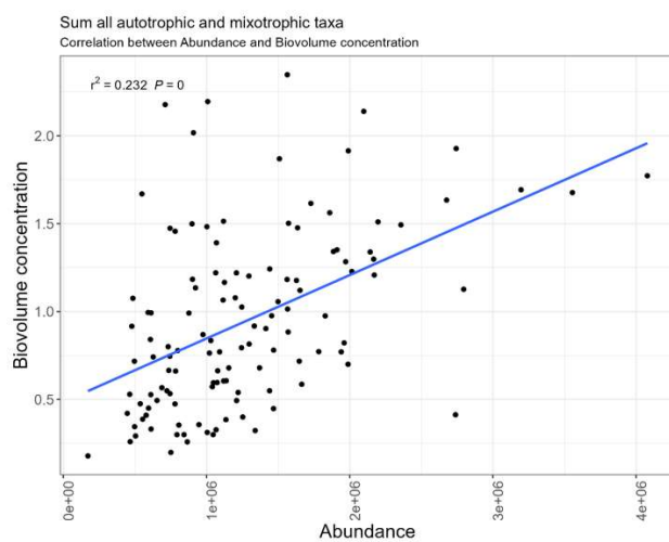
Fig. 16. Korrelation mellan celltäthet (cells L-1) och biovolym (mm 3 L-1)
