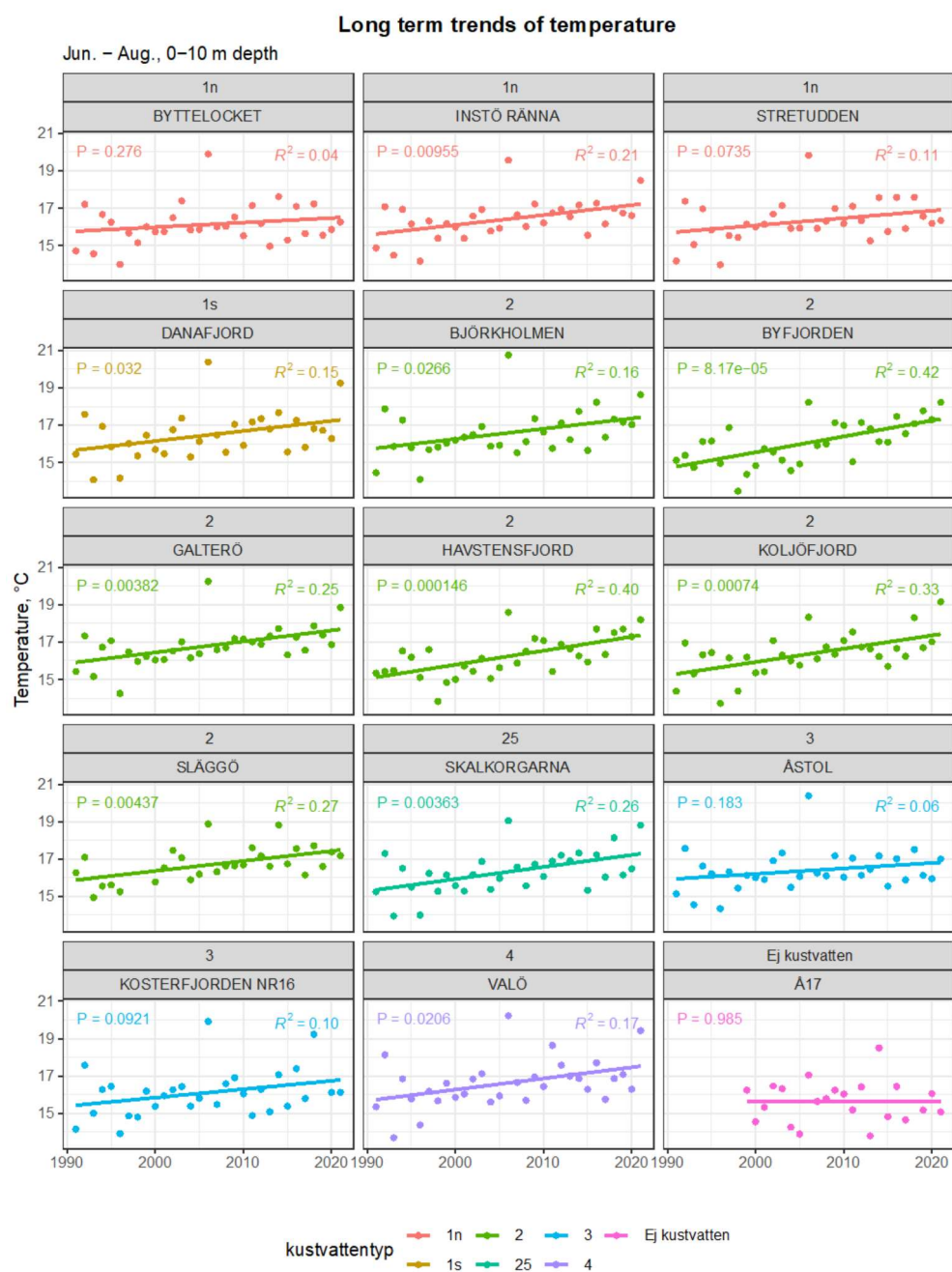
Fig. 41. Ytvattentemperatur sommartid för åren 1991–2021. Punkterna representerar medelvärden för mätningar i juni-augusti för respektive år. Linjär regression har använts för att anpassa linjer till värdena. P-värden <0,05 betraktas som signifikanta. R 2 värden visas också (se material och metoder).
