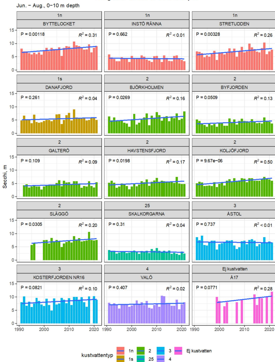
Fig. 28. Tidsserie för sommarmedelvärden för siktdjup vid 14 stationer längs Västra Götalands kust samt vid station Å17 i centrala Skagerrak. Den blå linjen representerar korrelation beräknad med linjär regression. P-värden <0,05 betraktas som signifikanta. R 2 värden ger ett mått på osäkerhet, se material och metoder. Siktdjup beror på en kombination av mängd växtplankton, mängd andra partiklar (bl.a. suspenderat sediment) och vattnets CDOM-halt (CDOM = Coloured Dissolved Organic Matter, bl.a. humus). Sommarmedelvärden 0–10 m djup för juni–augusti för perioden 1991–2021 visas. Station Å17 besöks ofta nattetid eller när solen står lågt. Då kan siktdjup inte mätas.
