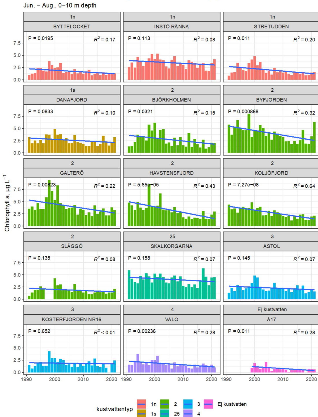
Fig. 26. Tidsserie för sommarmedelvärden för klorofyll a vid 14 stationer längs Västra Götalands kust samt vid station Å17 i centrala Skagerrak. Den blå linjen representerar korrelation beräknad med linjär regression. P-värden < 0,05 betraktas som signifikanta. R^2 värden ger ett mått på säkerhet, se material och metoder. Klorofyll a är ett grovt mått på växtplanktonbiomassa. Sommarmedelvärden 0–10 m djup för juni–augusti för perioden 1991–2021 visas.
