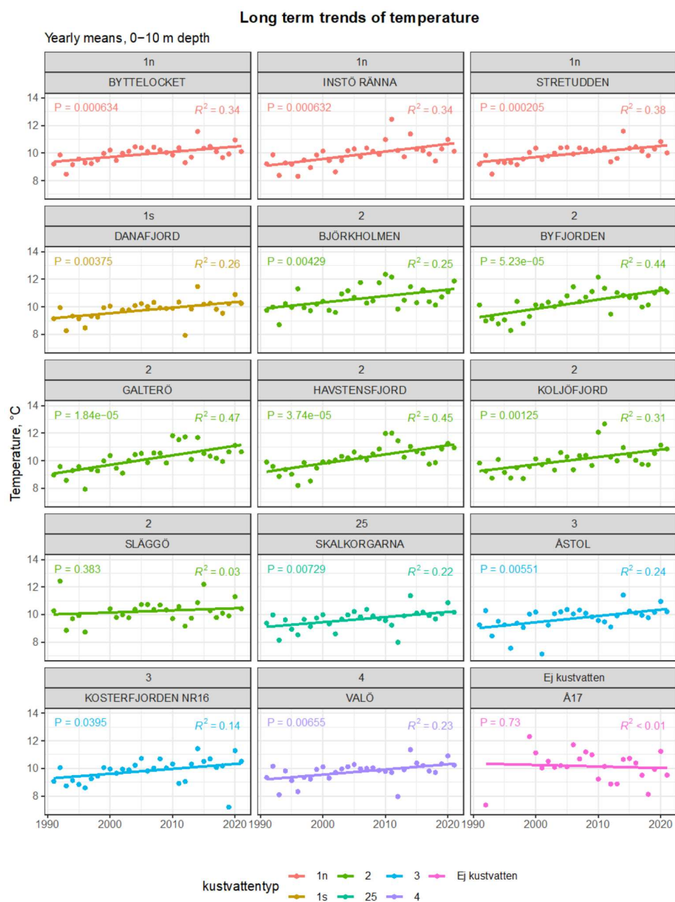
Fig. 40. Ytvattentemperatur, årsmedelvärden för åren 1991–2021. Punkterna representerar medelvärden för mätningar alla månader respektive år. Linjär regression har använts för att anpassa linjer till värdena. P-värden <0,05 betraktas som signifikanta. R 2 värden visas också (se material och metoder).
