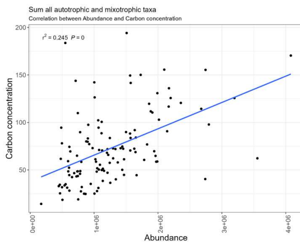
Fig. 17. Korrelation mellan celltäthet (cells L-1) och biomassa (µg C L-1)
