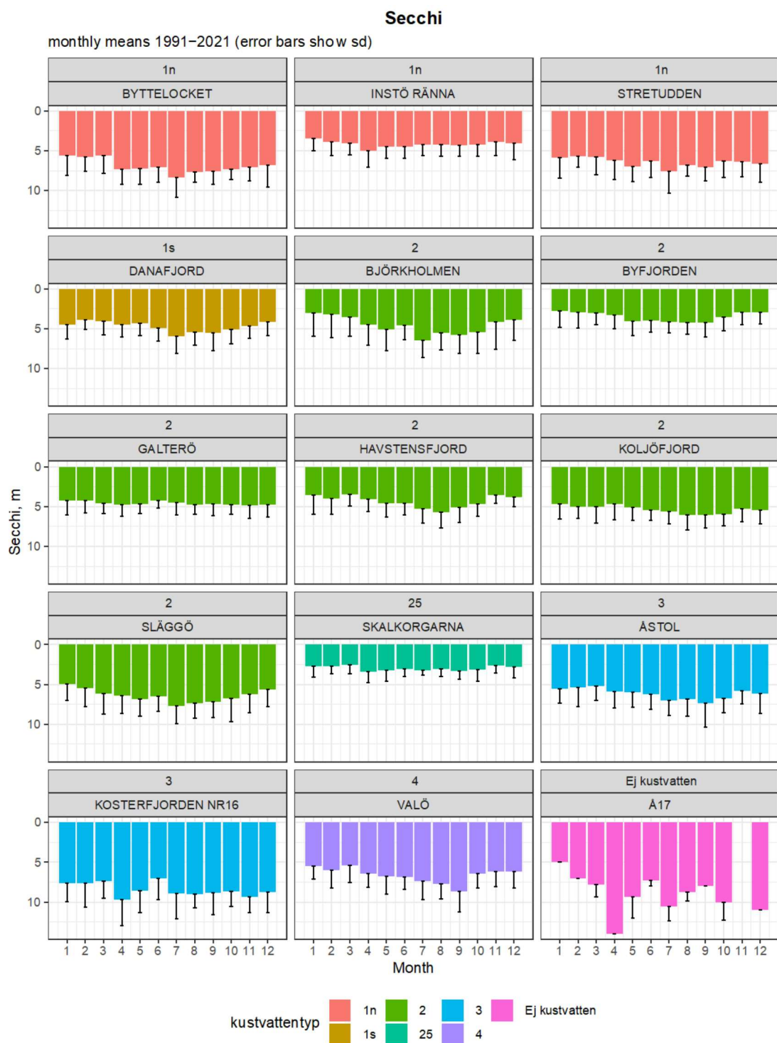
Fig. 27. Månadsmedelvärden för siktdjup vid 14 stationer längs Västra Götalands kust samt vid station Å17 i centrala Skagerrak. Siktdjup beror på en kombination av mängd växtplankton, mängd andra partiklar (bl.a. suspenderat sediment) och vattnets CDOM-halt (CDOM = Coloured Dissolved Organic Matter, bl.a. humus). Medelvärden ( \pm en standardavvikelse) för 0–10 m djup för perioden 1991–2021 visas. Notera att antal mätningar vid Å17 är lägre än på andra stationer. Stationen besöks ofta när det är mörkt eller när solen står lågt vilket omöjliggör siktdjupsbestämning.
