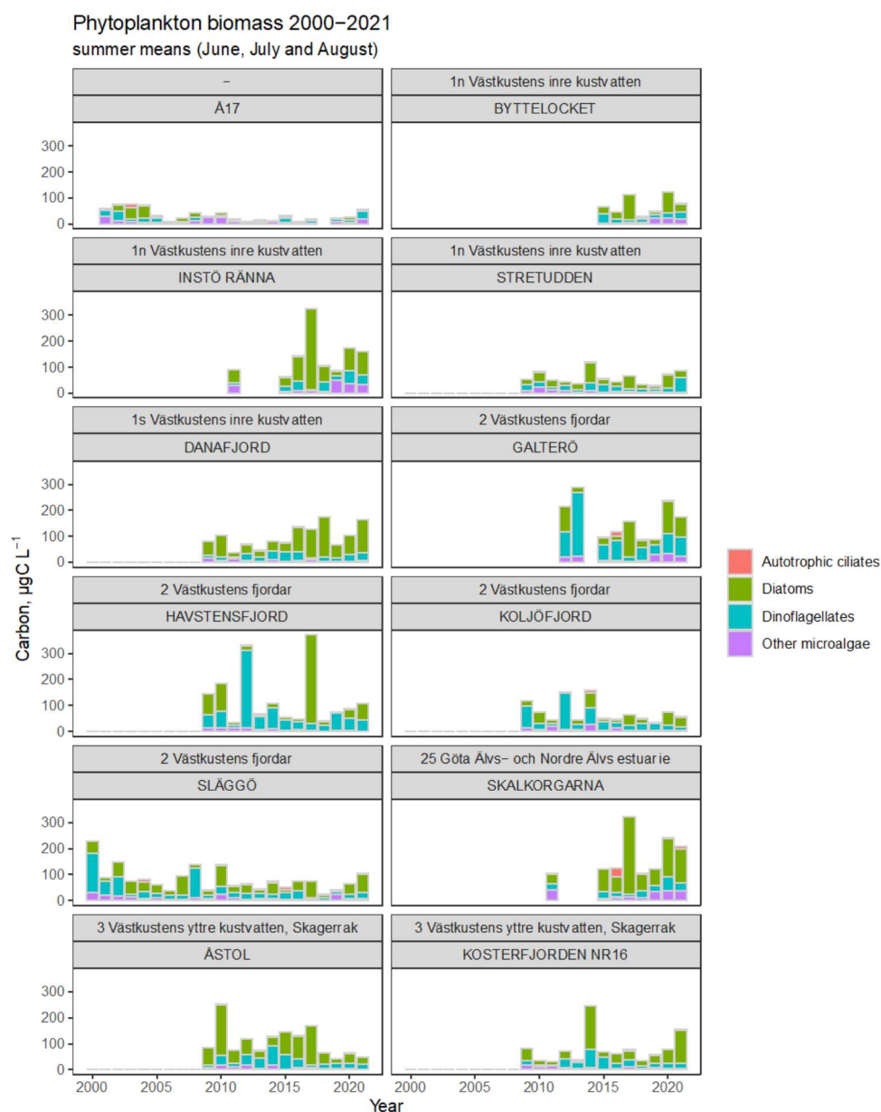
Fig. 10. Sommarmedelvärden för växtplanktonbiomassa (enhet i kol) vid tolv stationer. Biomassan är uppdelat i huvudgrupper av växtplankton. Mätningar av biomassa påbörjades år 2000 vid Släggö, år 2001 vid Å17 och år 2009 vid BVVF-stationerna. Vid fyra stationer som finansieras av Länsstyrelsen för Västra Götaland startade mätningarna ca år 2016. Åren 2011 genomfördes en mätkampanj då ovanligt många stationer provtogs.
