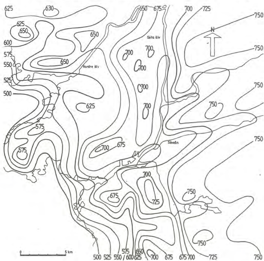
ÅRSNEDERBÖRD 1978 från analys i kartskalen 1:3·10 6
